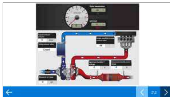
SYSTEME DE DOSAGE DE L'AGENT REDUCTEUR.
